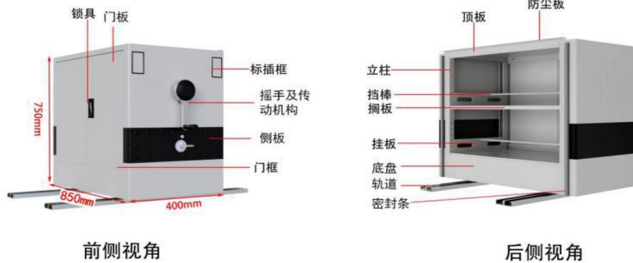
成型密集架小样结构效果图
